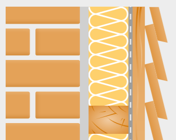
Vertikalschnitt: waagerechte Stülpeschalung
