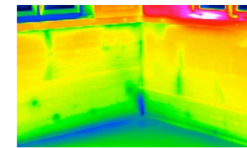
Abbildung 20 Thermografieaufnahme nach 20 s bei 50 Pa Unterdruck
