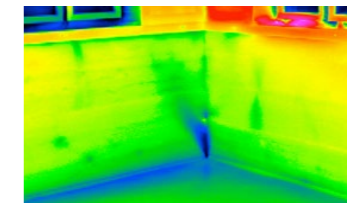
Abbildung 21 Thermografieaufnahme nach 300 s bei 50 Pa Unterdruck
